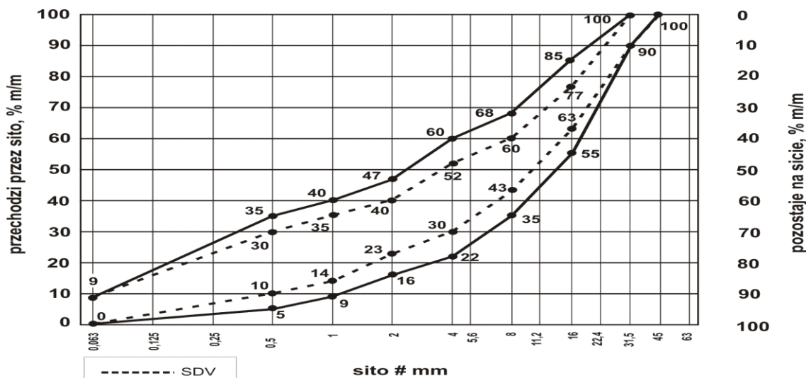
Rys. 1. Uziarnienie mieszanki niezwiązanej 0/31,5 dla podbudowy zasadniczej oraz warstwy ulepszanego podłoża
