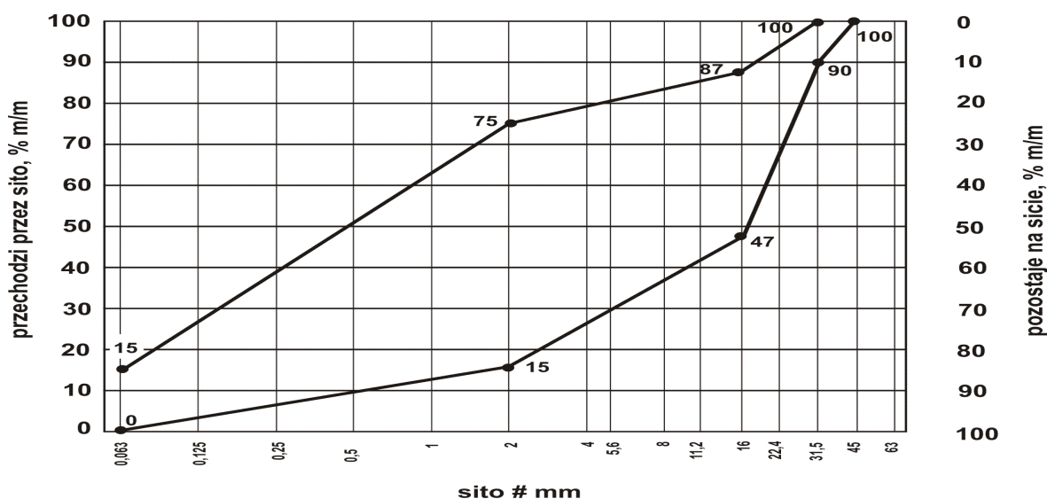
Rys. 2. Uziarnienie mieszanki niezwiązanej 0/31,5 dla nawierzchni (nawierzchnie zjazdów z kruszywa i poboczy)
